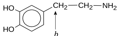
la dopamine
