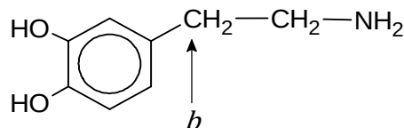
dopamina
