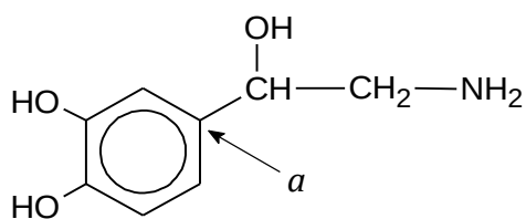
норадреналин
